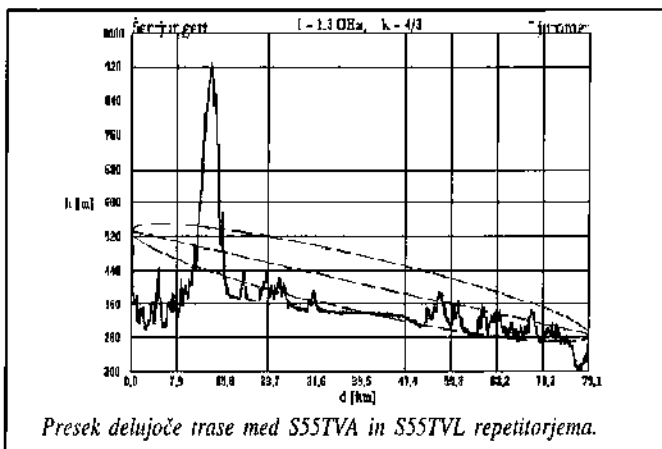
Za link povezavo potrebujemo višje frekvenčne pasove, saj so na obeh straneh izhodi repetitorjev na 23cm. "Preboj" Konjiške gore je na 23cm
